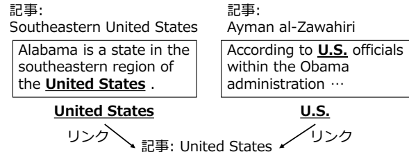
図 1: 擬似的な共参照データの生成に用いる Wikipedia の内部リンク.
