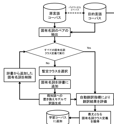
図2 データ構築処理
