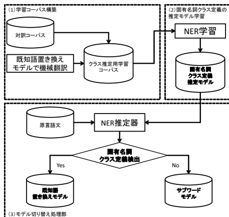
図1 提案手法の処理概要
